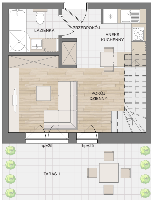
POZIOM 0
